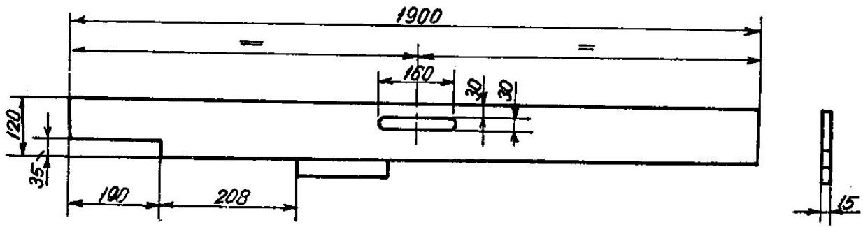
Fig.16 Șablon pentru montarea și verificarea gabariturii inductoarelor de cale
