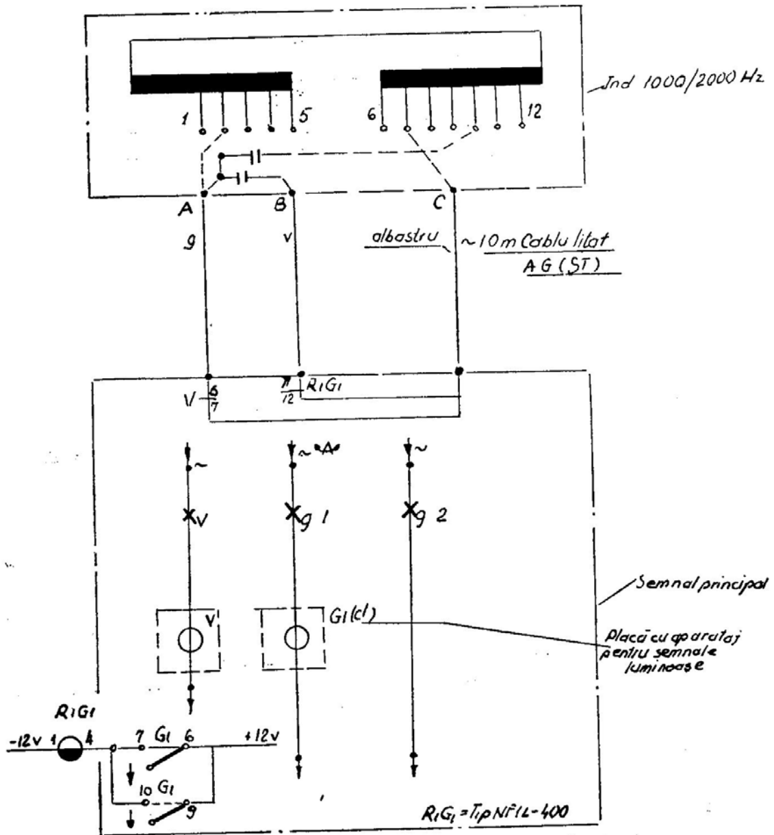
Fig. 68 Schema electrică și conectarea la semnalul de ieșire, alimentat în curent continuu de la linia directă, pe secții cu B.L.A., cu galben-clipitor
