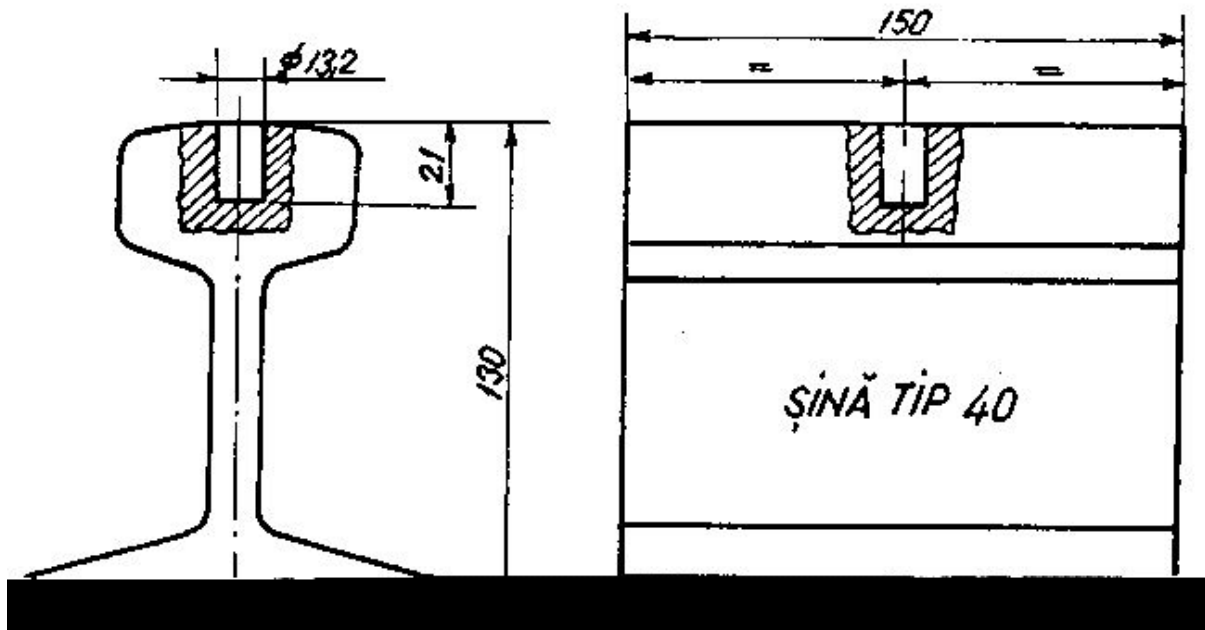
Fig. 24 Piesă pentru nituirea bolțului la contactoare
