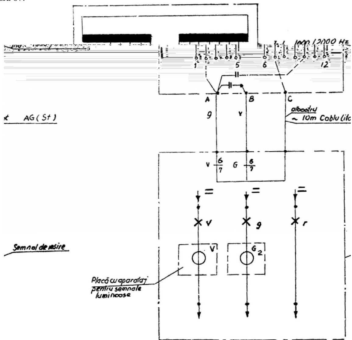
Fig. 66 Schema electrică și conectarea la semnalul de ieșire, alimentat în curent continuu, de la linia directă pe secții cu B.L.A.
