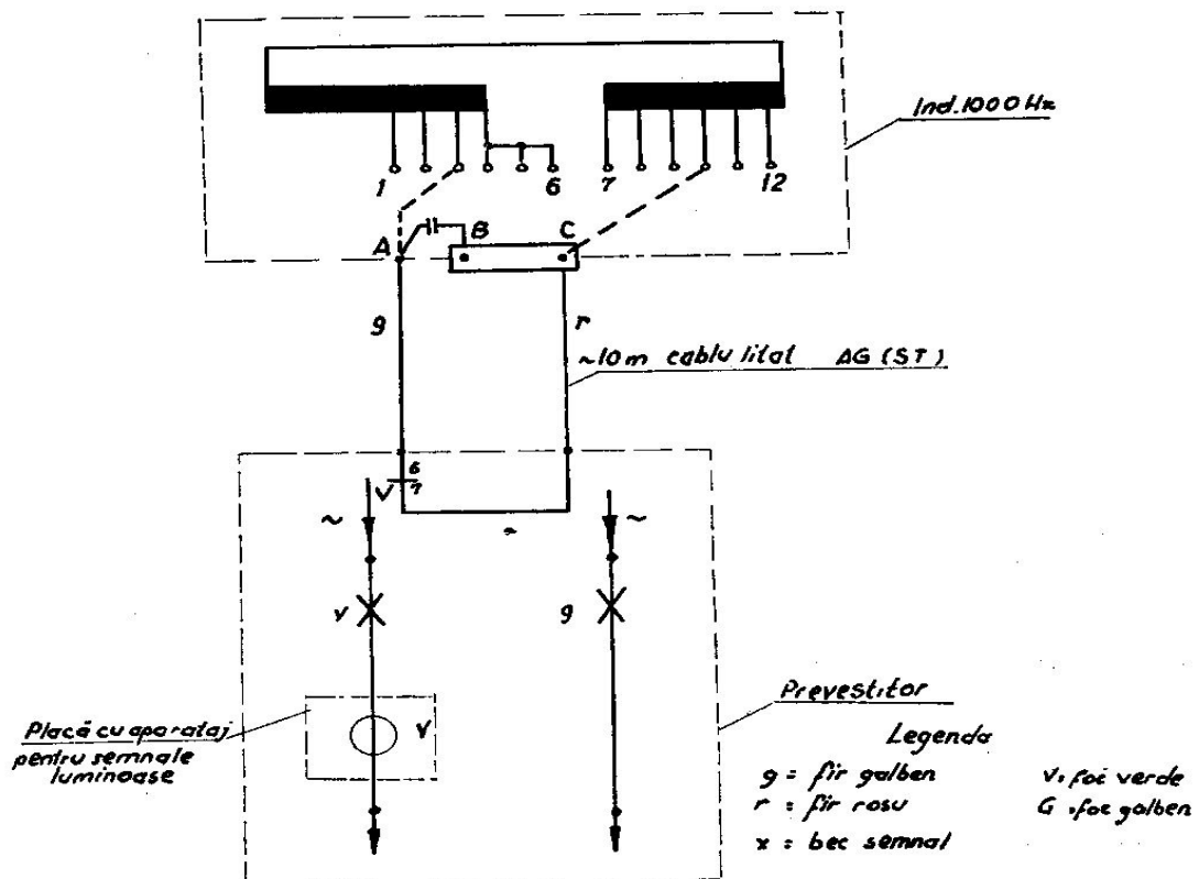
Fig. 47 Schema electrică și conectarea la semnalul prevestitor pe secții fără BLA, echipat cu inductor de cale de 1000 Hz
