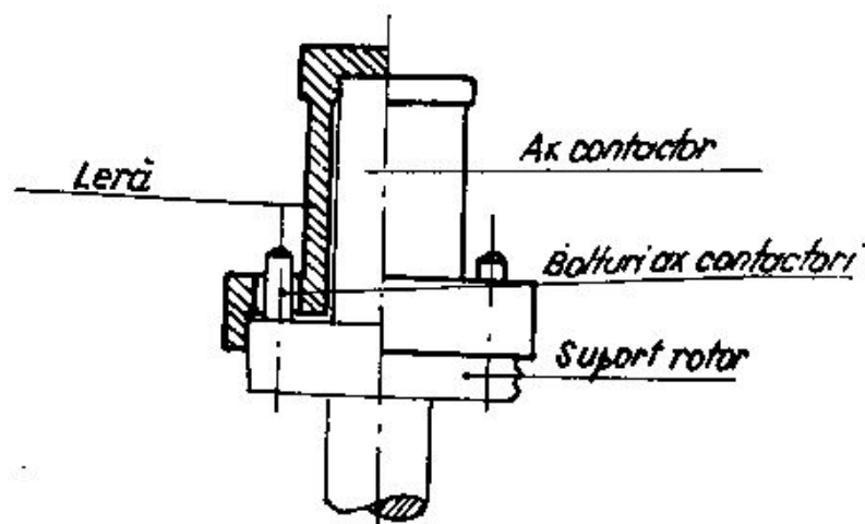
Fig. 22 Lera pentru reglajul poziției axului contactorului
