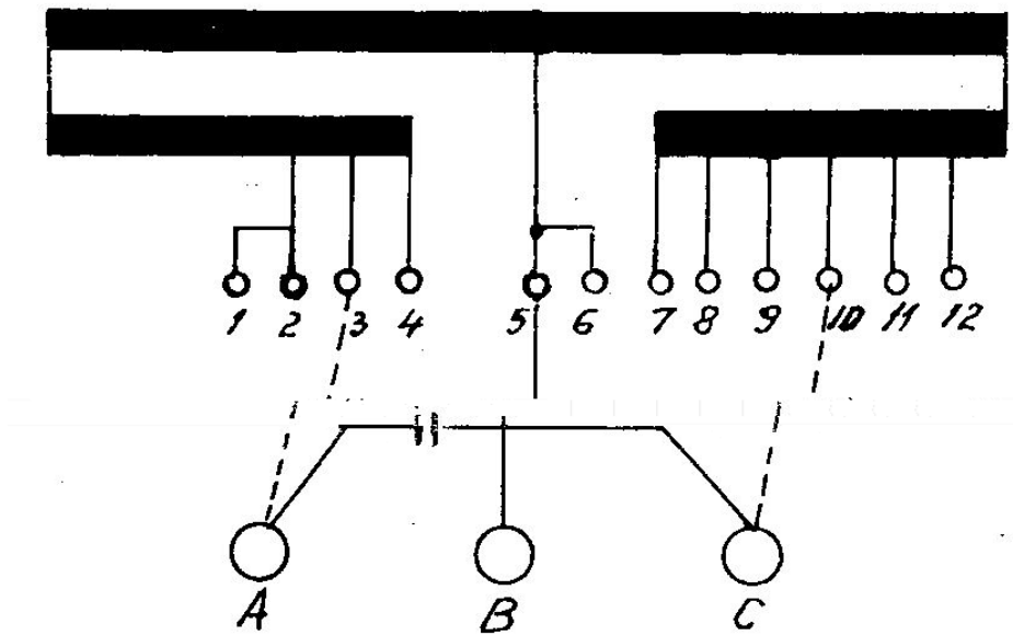
Fig. 7 Conexiuni electrice la inductorul de cale de 500 Hz
