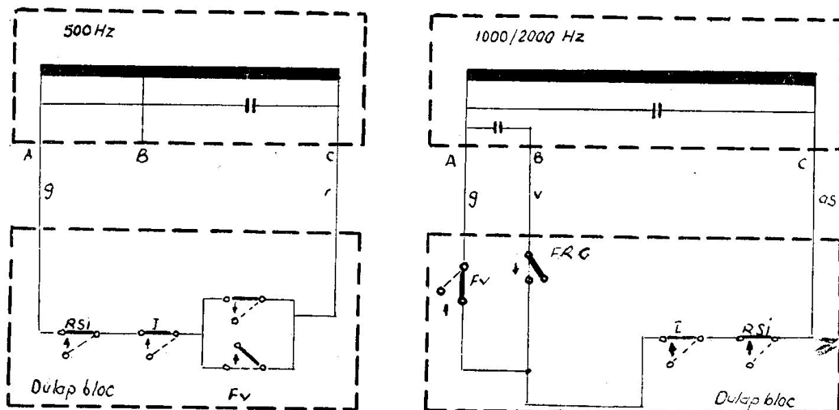
Fig. 52 Conectarea inductoarelor de cale la semnalul prevestitor pe secții cu B.L.A. în curent continuu, cu două relee de foc, prin utilizarea de contacte ale releelor din schema blocului de linie
