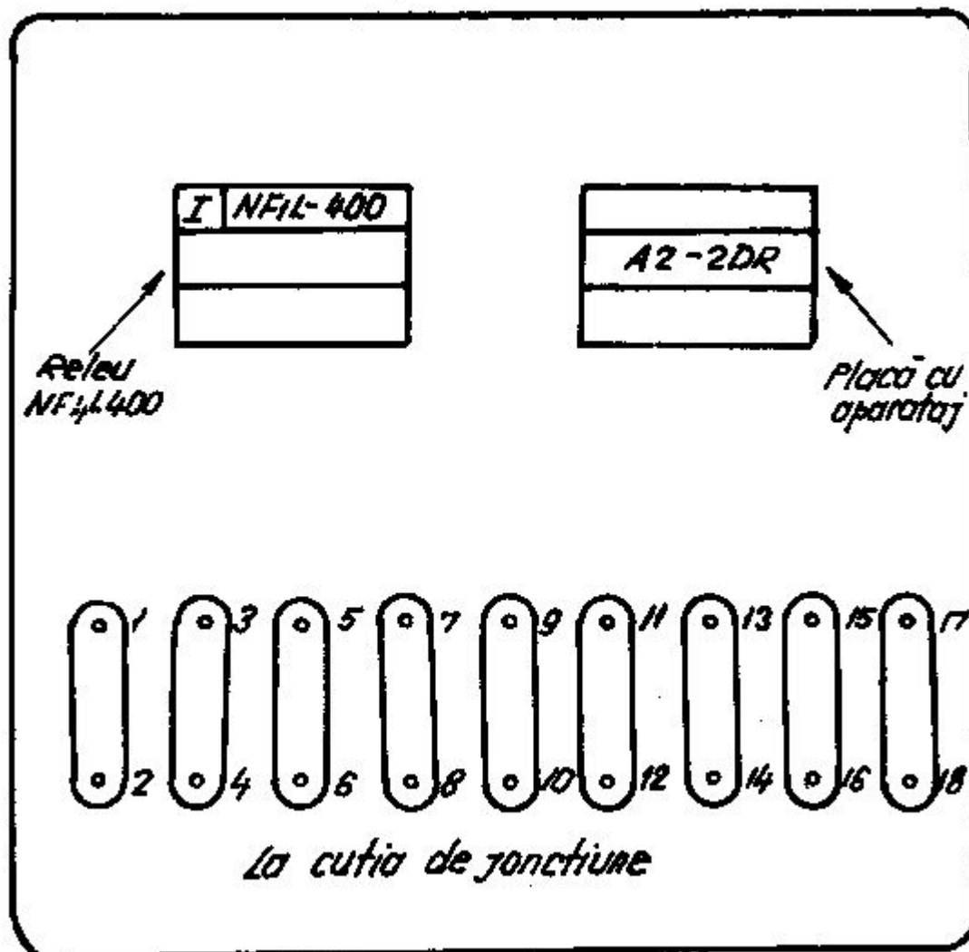
Fig. 30 Montarea plăcii cu aparataj și a releului NF1L-400 în pichetul PA-1
